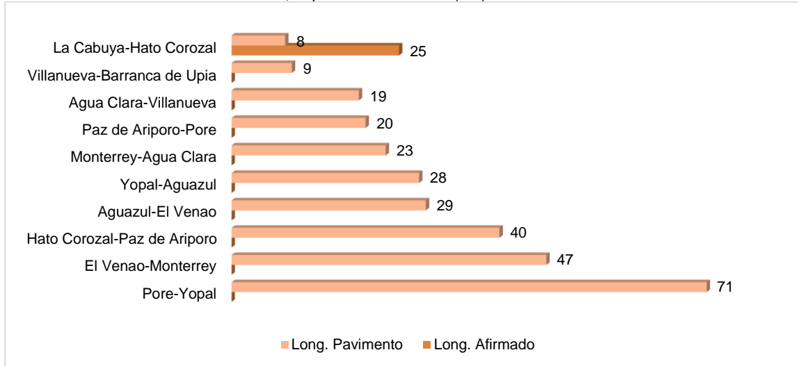
Gráfica 216. Red de Vías Troncal del Llano, Superficie de Rodadura (Km) 2016.
